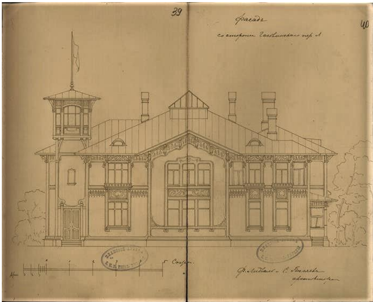
Del av bygglovsansökan för Ekvalls bostadshus. Arkitekt: Fredrik (Fjodor) Lidvall.
